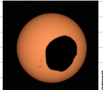
フォボスによる火星の日食 April 20, 2022
